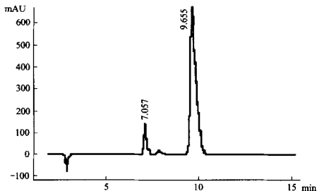
图 2 试样中唑禾灵 R、S 对映体拆分色谱图
