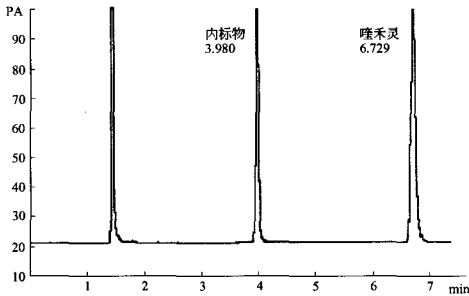
图 1 精啶禾灵原药与内标物气相色谱图
