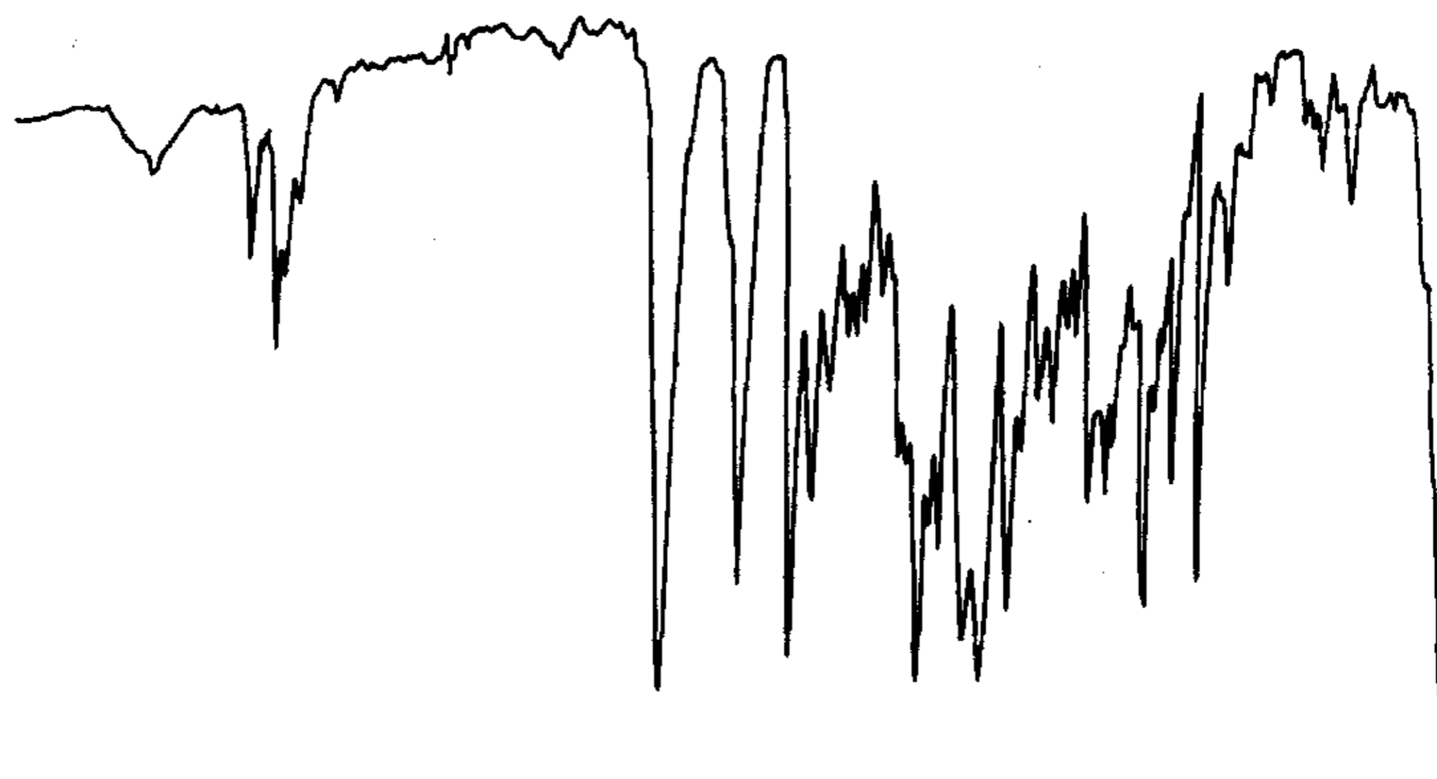
图 1 氯氰菊酯标准品的红外光谱图
